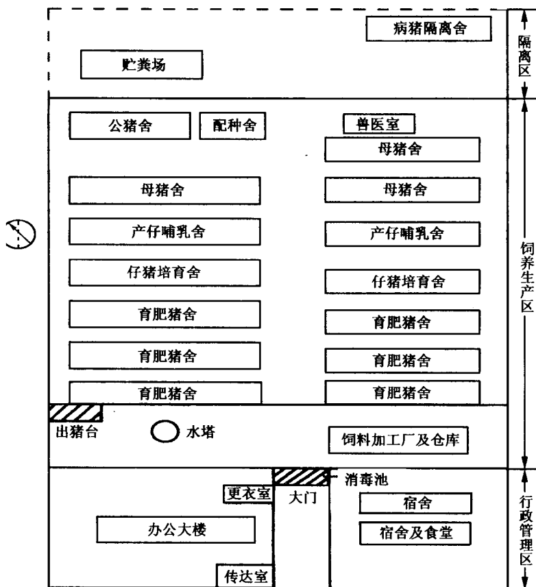
图 1-1 一般猪场平面布局示意图
