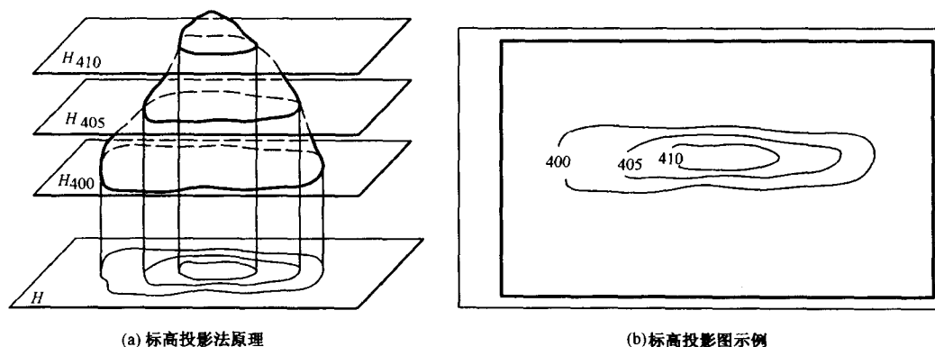
图 1-6 标高投影法与地形图
