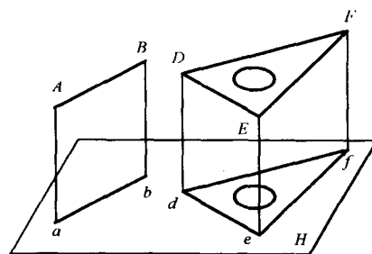
图 1-9 显实性 (实形性)
