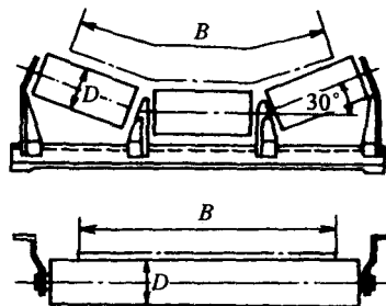
图 2-2 托辊结构示意图
