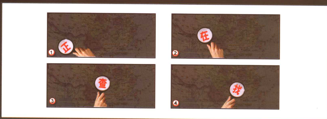
图 13-34 查找动画
