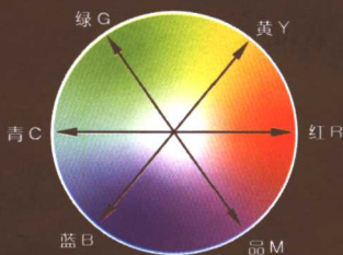
图 4-1 色轮图
