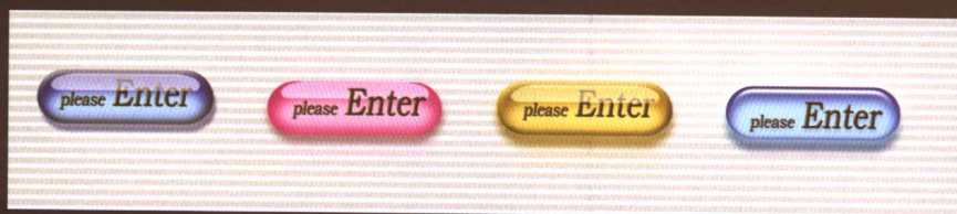
图 7-131 玻璃按钮
