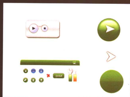
图 14-69 按钮
