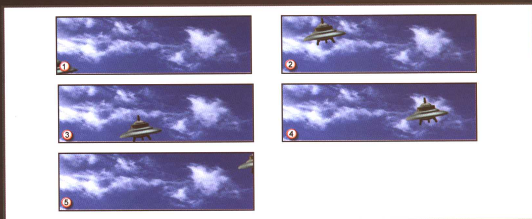
图 13-19 飞行动画
