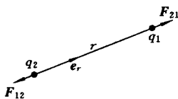
图 9-1-1 库仑定理
