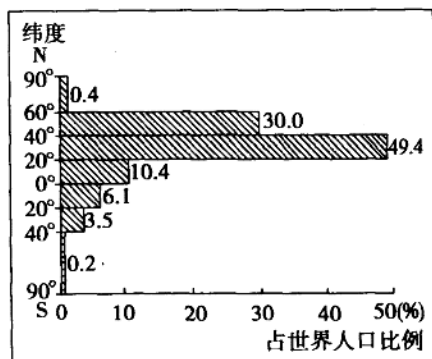
图二 世界人口纬度分布
