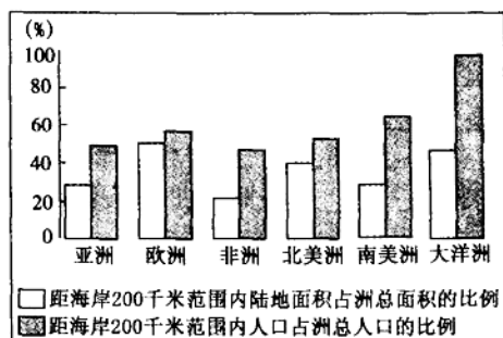
图三 世界大洲海岸 200 千米范围内陆地面积、人口占洲总面积、总人口的比例
