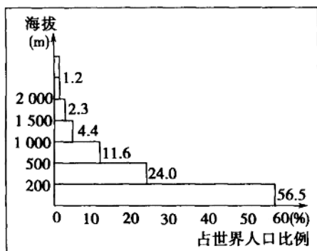
图一 世界人口垂直分布
