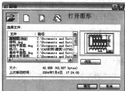
图 1-2 “启动”对话框
