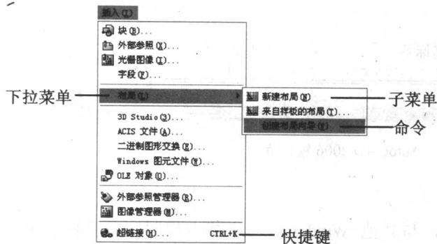
图 1-7 下拉菜单
