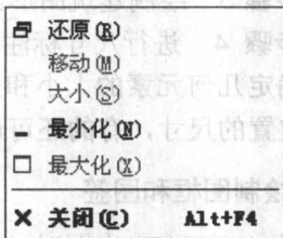
图 1-4 快捷菜单
