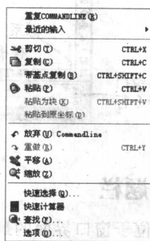
图 1-8 快捷菜单
