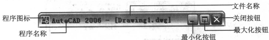
图 1-6 标题栏
