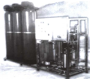
反渗透设备（每小时处理水量为0.5吨）
