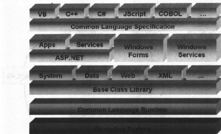
图 1-1 .NET Framework
