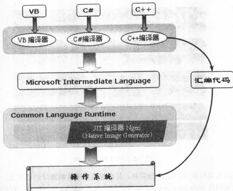
图 1-2 基于 CLR 的代码的运行步骤
