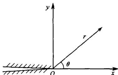
图 0.1-1 裂纹顶端与坐标系
