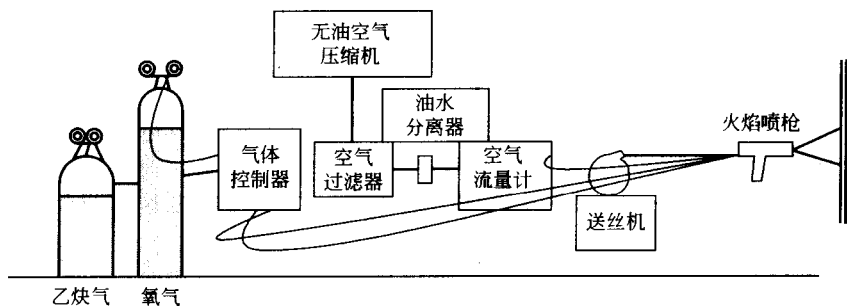
图 1-5 典型的火焰喷涂系统示意图
