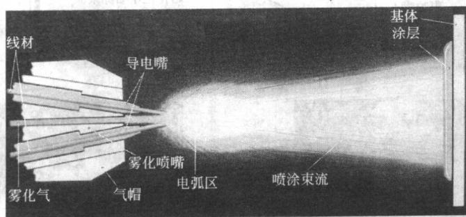
图 1-11 电弧喷枪工作原理示意图
