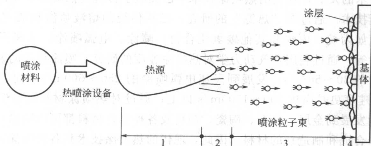
图 1-1 热喷涂原理示意图
