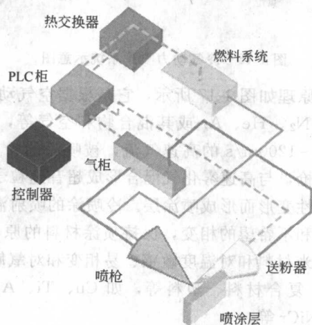
图 1-14 高速火焰喷涂系统的示意图
