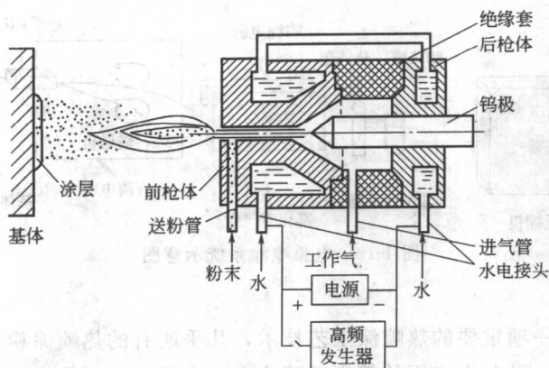
图 1-13 等离子喷枪工作原理示意图
