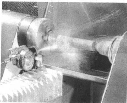
图 1-8 线材火焰喷枪喷涂实例图
