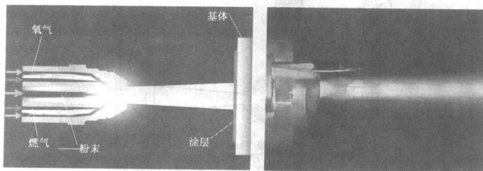
图 1-15 高速火焰喷枪工作原理示意图（右图为 HVOF 喷涂示例）
