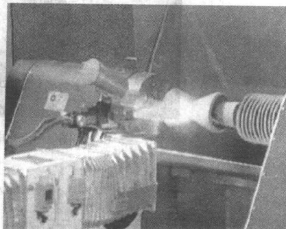
图 1-9 粉末火焰喷枪喷涂实例图
