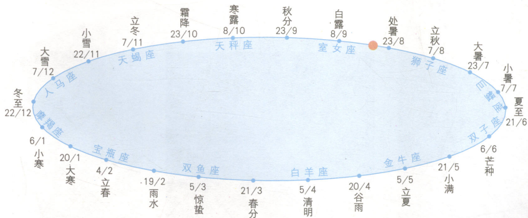
黄道上二十四节气点、阳历日期和黄道十二星座的配置关系
