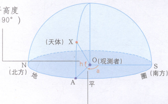
天体的地平坐标
