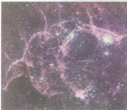
船帆座超新星遗迹和脉动星
