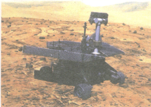
在火星表面的“勇气号”
