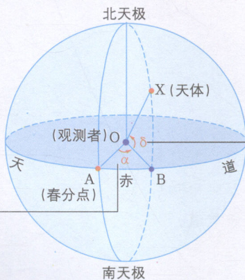
天体的赤道坐标
