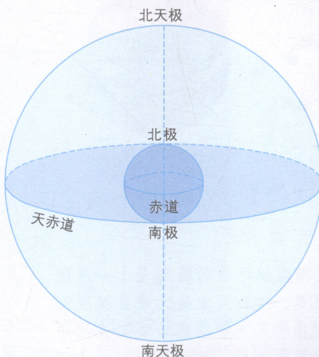
天球上的天极和天赤道
