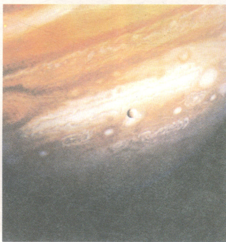
“旅行者1号”拍摄的木星
