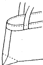
B 面料布和衬里布各自缝成袋状后， 套在一起再缝去包角
