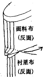
C ①把面料布袋和衬里布袋从 底部相对，缝去包角
