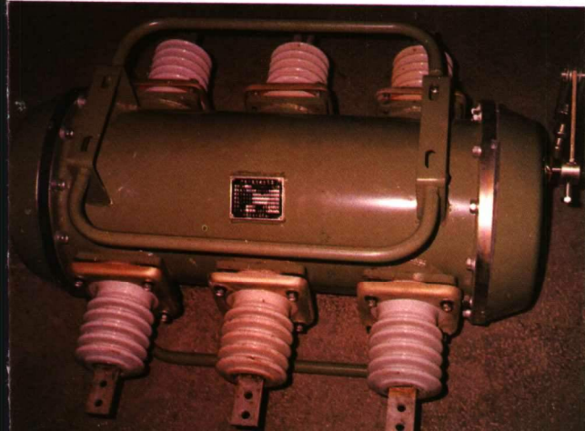
电器设备厂产品——六氟化硫断路器
