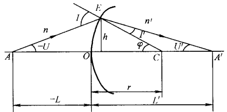
图 1-10 光线经过单个折射球面的折射
