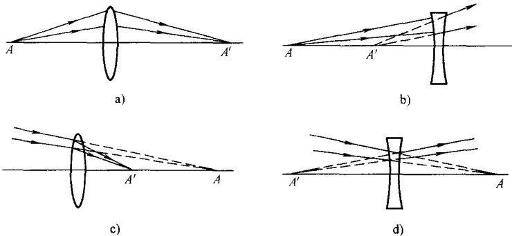
图 1-9 物、像的虚实
