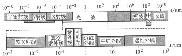
图 1-1 电磁波谱
