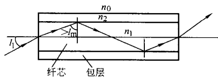
图 1-6 光纤的全反射传光原理
