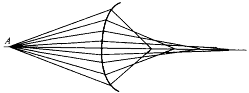
图 1-11 轴上点成像的不完善性
