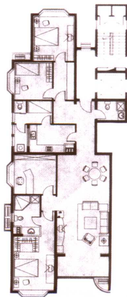
平面图
