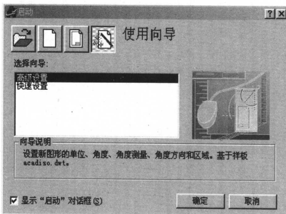
图 2-1 【启动】对话框
