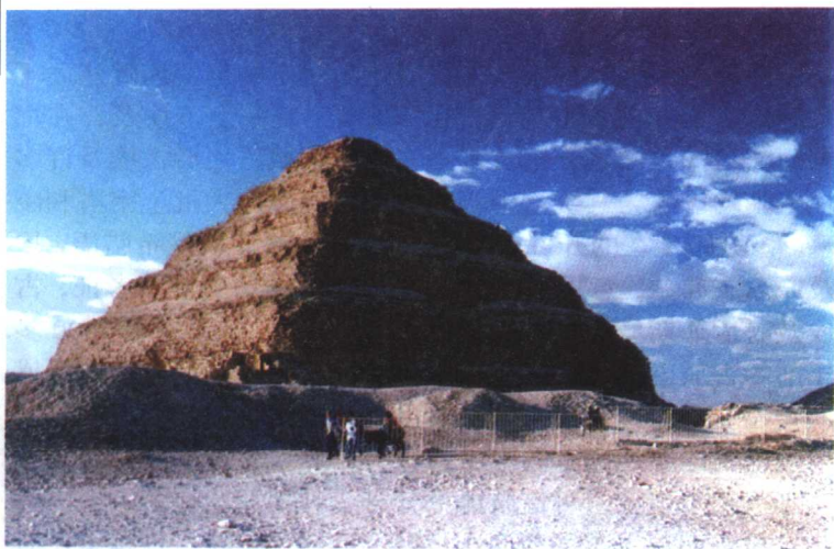
梯形金字塔
