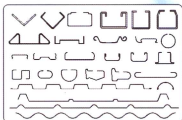
Metal sheet forming section 金属板件成型断面图
