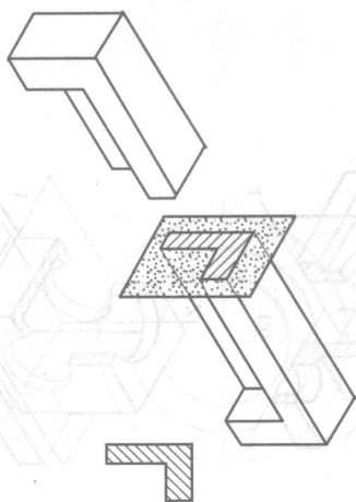
图 1-17 剖面图
