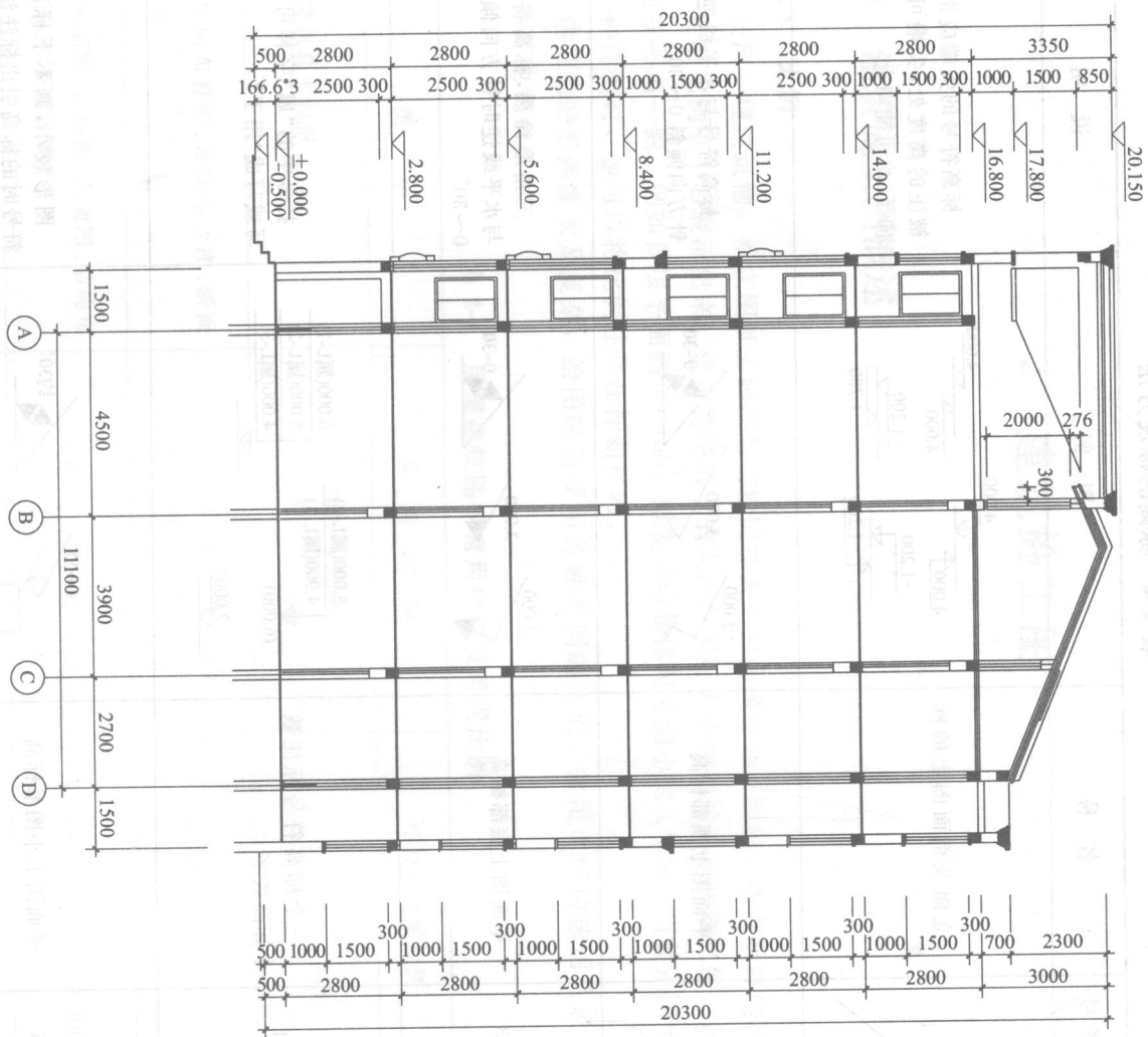
图 2-3 相对标高
