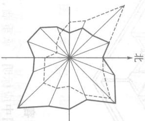
图 2-10 风玫瑰
