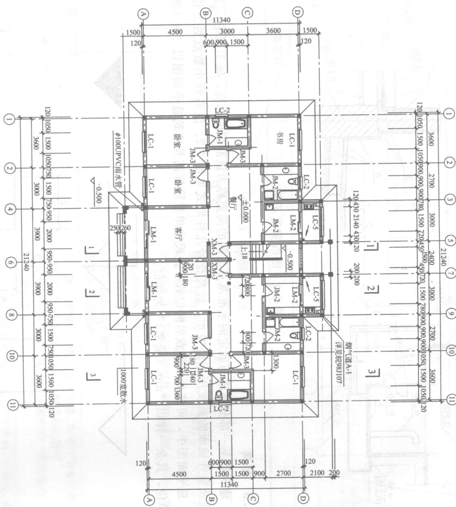
图 2-4 定位轴线
