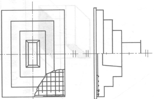
图 1-13 钢筋混凝土独立基础两面投影
