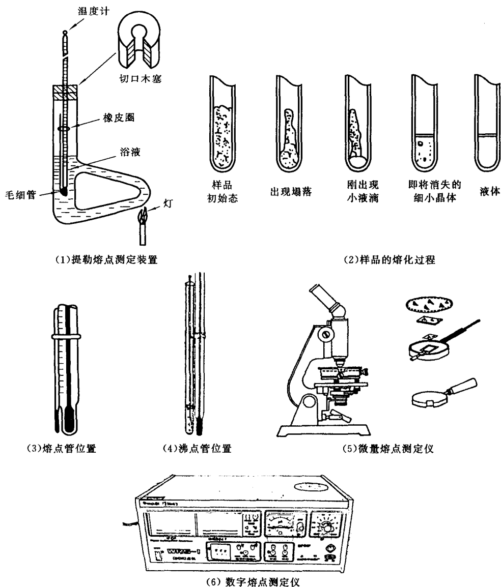
图 1-3 熔点(沸点)测定装置
