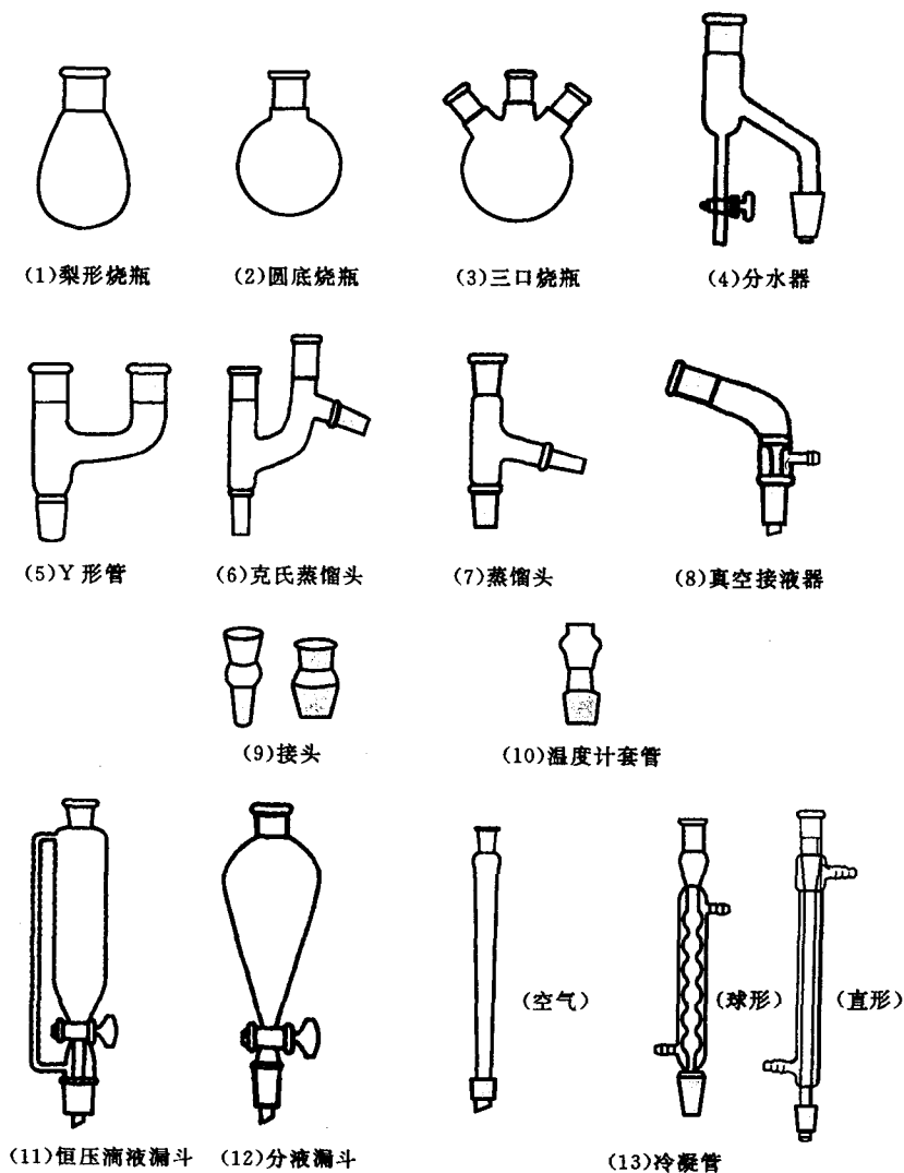
图 1-2 标准磨口玻璃仪器
