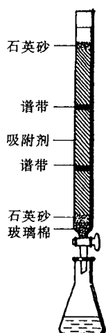
图 1-7 柱色谱装置
