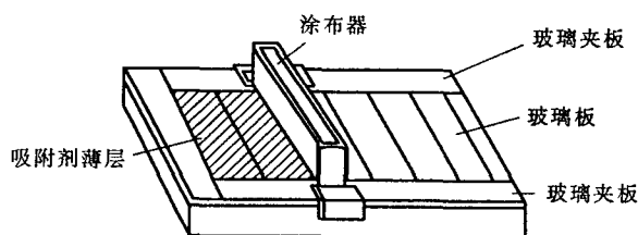
图 1-6 薄层涂布器
