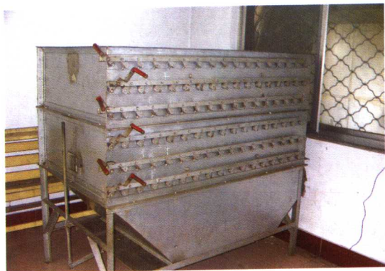
彩图 13 金银花茶叶加工的多层干燥箱（杀叶绿素之后干燥用）
