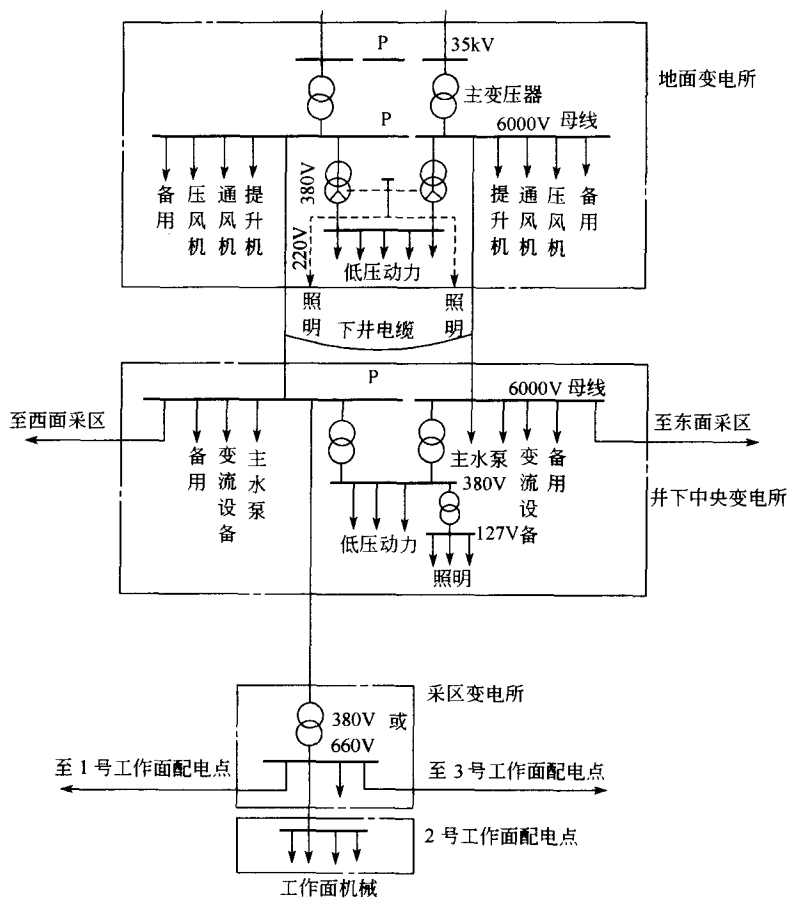
图 1-1 煤矿供电系统
