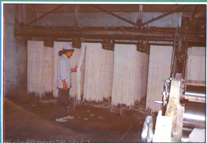
市粮油制品 厂挂面车间。
