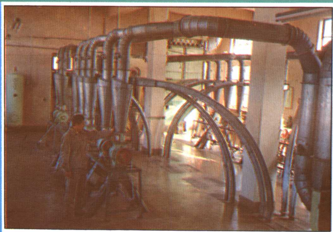
张家口 市面粉厂粉 间的风运设 备。
