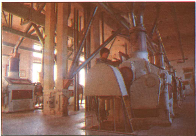
张家口市面粉 厂粉间正在运转的 磨粉机。
