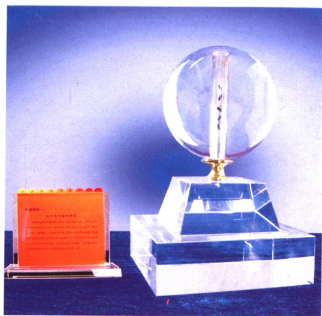
放置在水晶球内的八十垵 古稻谷，距今9000多年。
