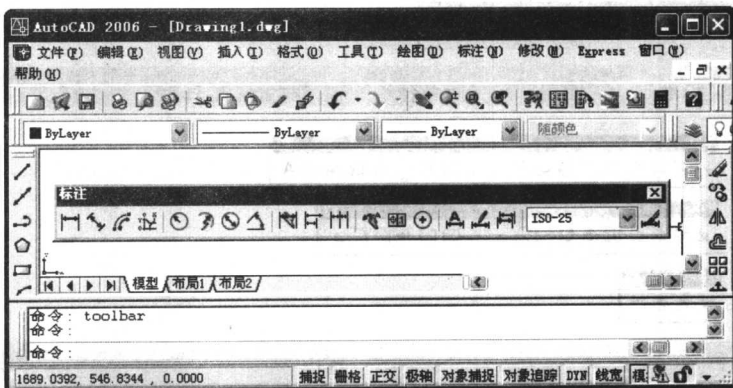
图 1-20 “浮动”工具栏
