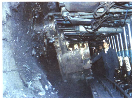
井下采煤机
