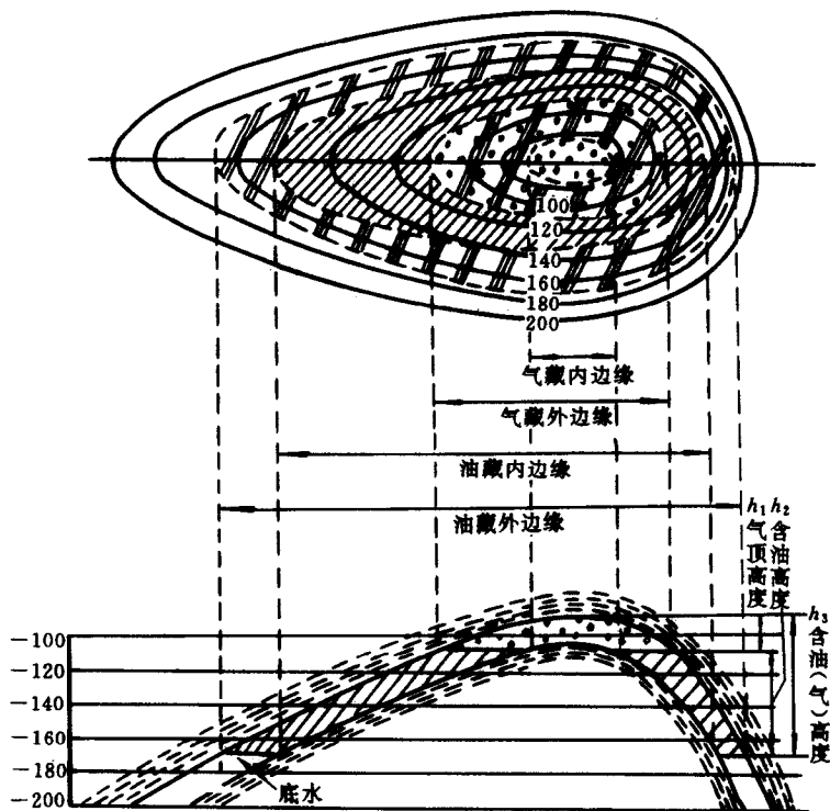
图 1-1 背斜油藏中油气水分布示意图
