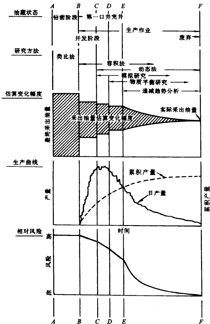
图 1-2 储量测算模式图
