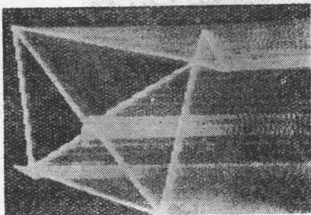
图3 由计算机模拟的光帆飞行情况
