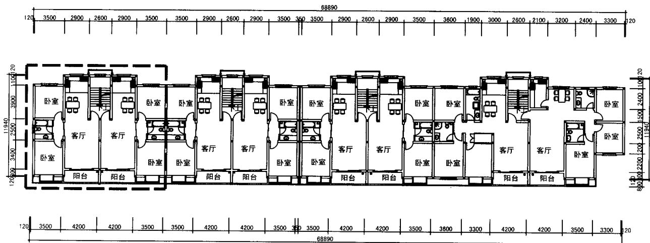
标准层平面图
