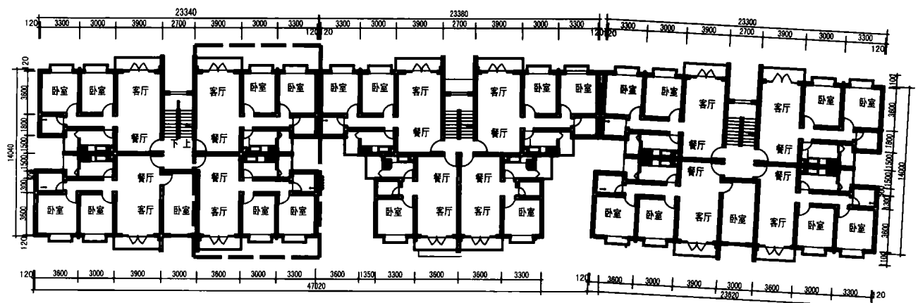
标准层平面图
