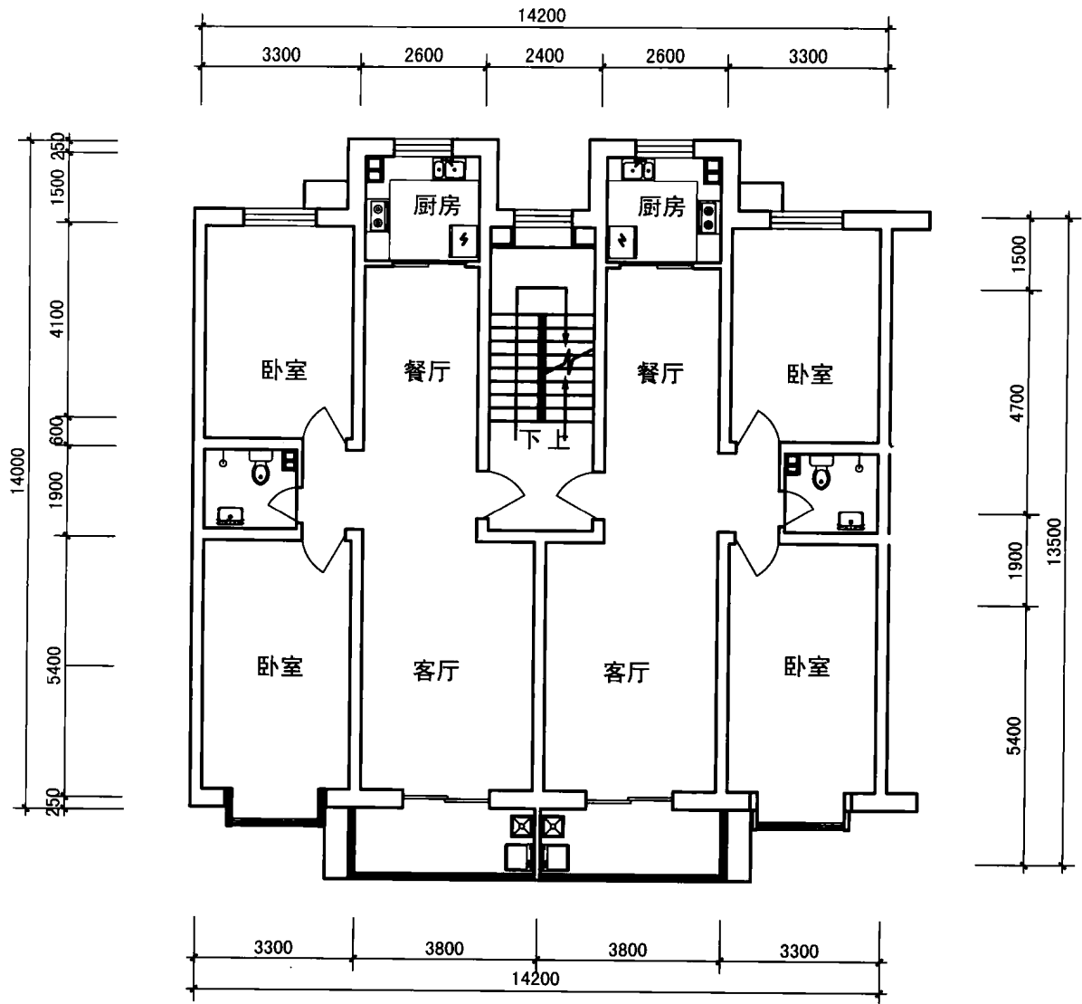
经典户型平面图
