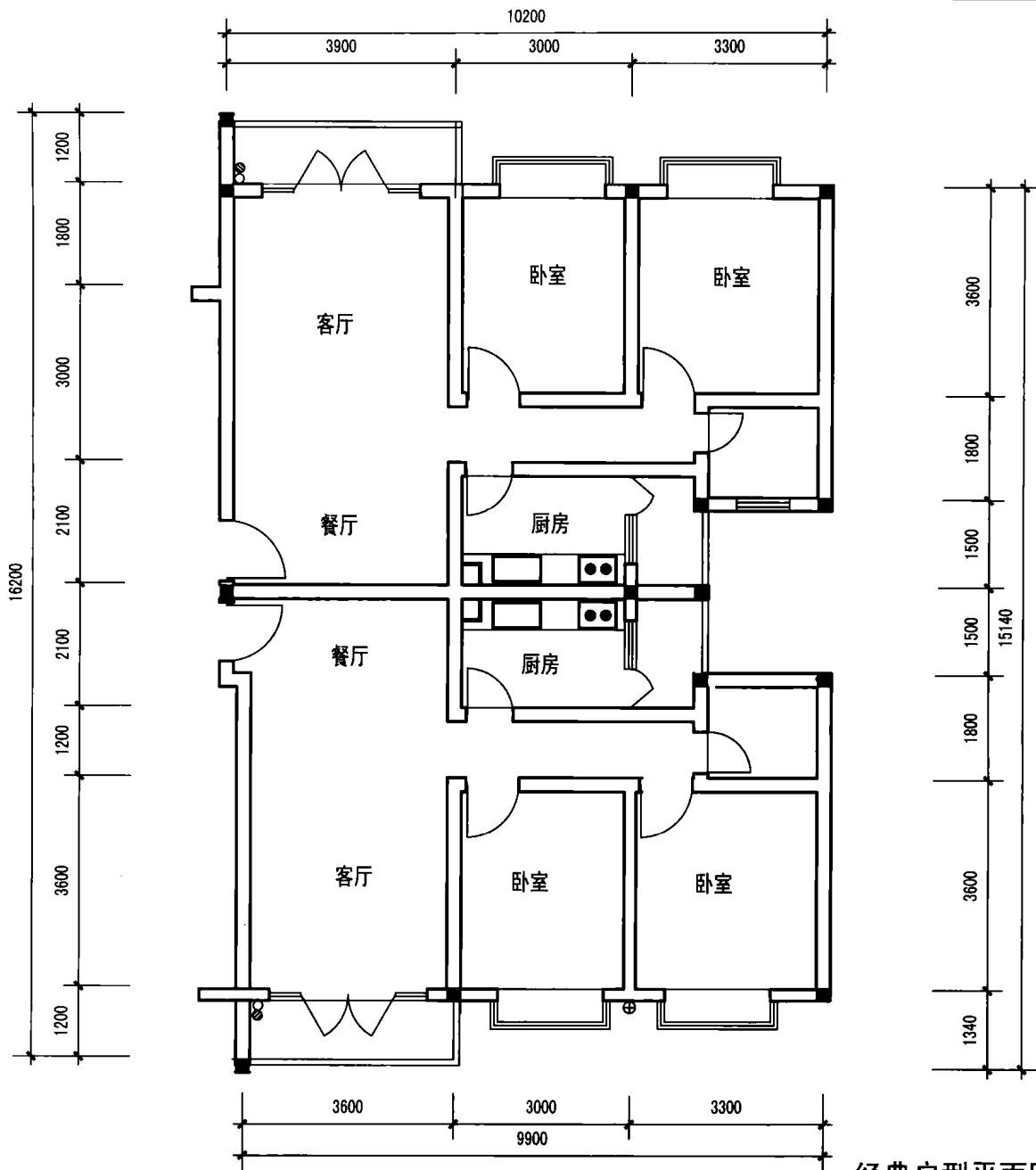
经典户型平面图
