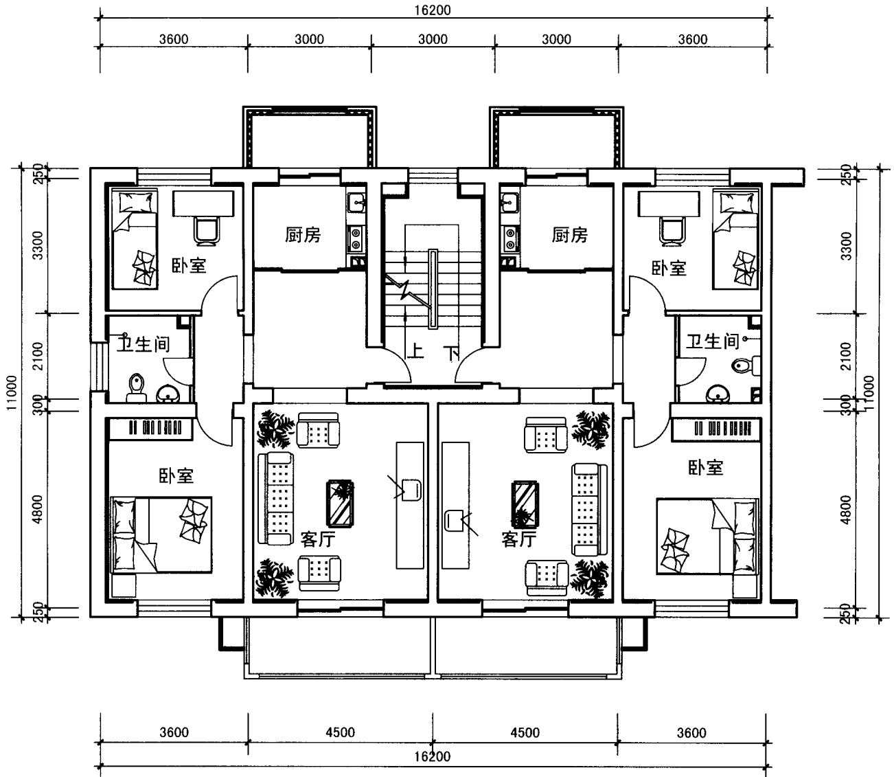
经典户型平面图
