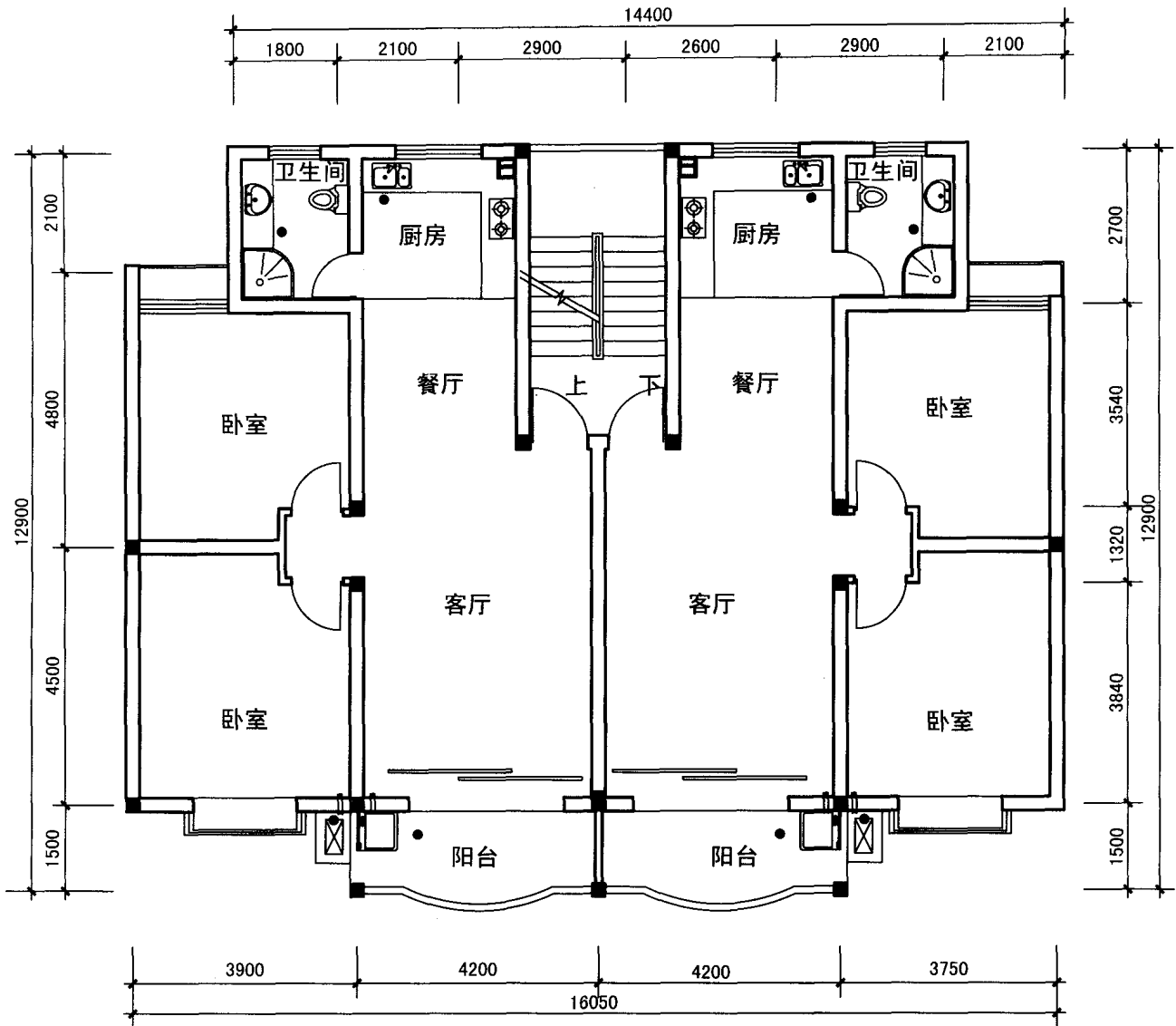
经典户型平面图
