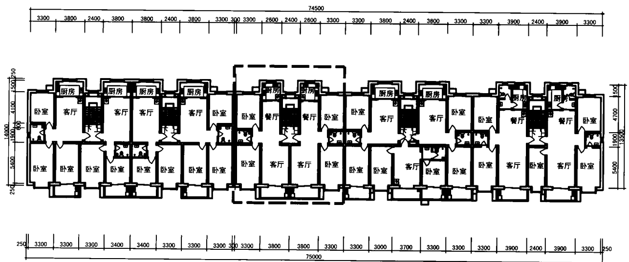
标准层平面图
