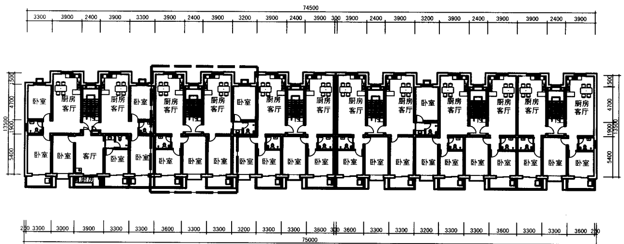
标准层平面图
