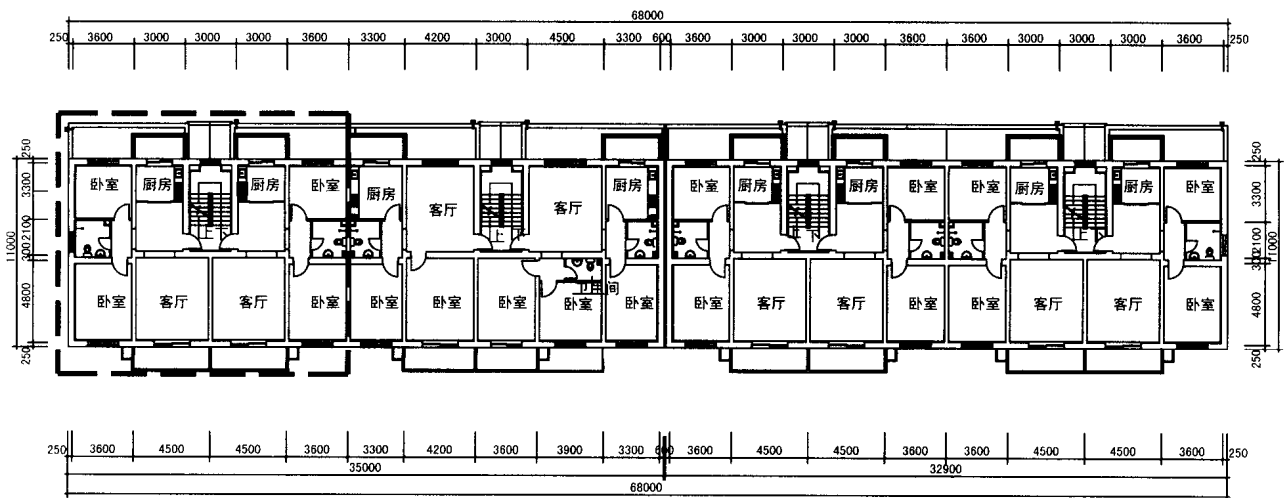
标准层平面图
