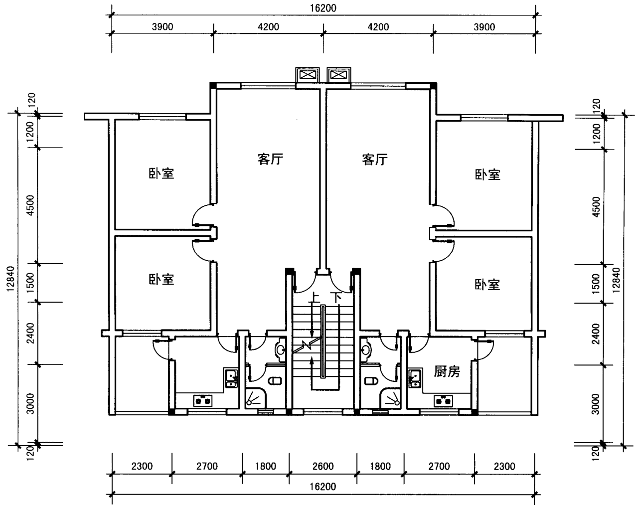
经典户型平面图
