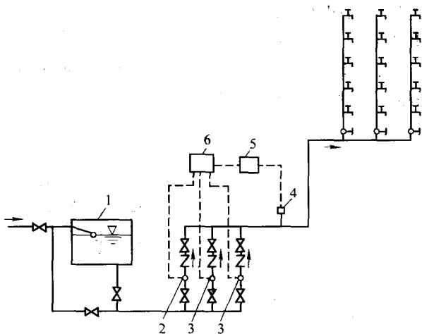
图 1-5 变速水泵供水方式
