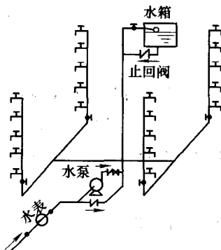
图 1-4 设置水泵和水箱给水方式
