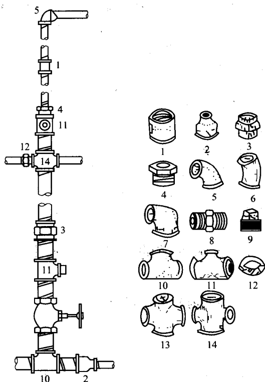
图 1-9 螺纹连接配件
