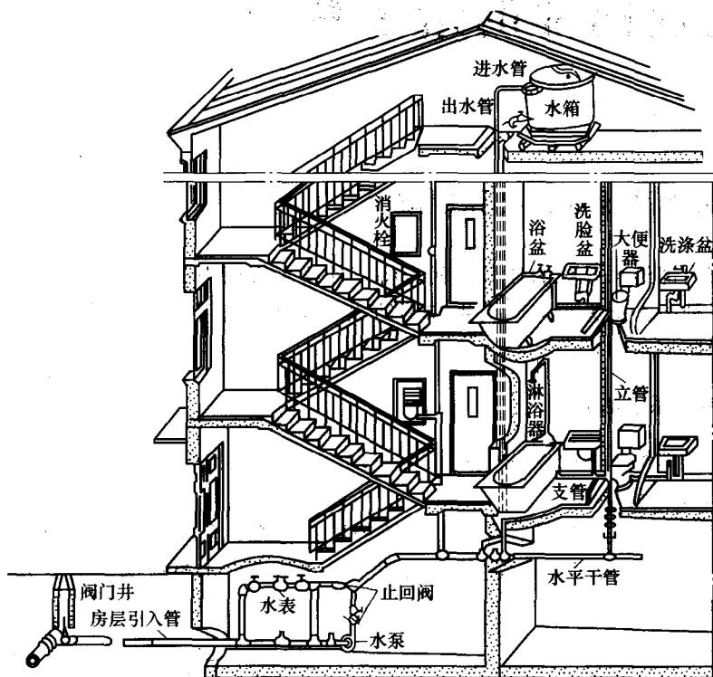
图 1-1 建筑内给水系统
