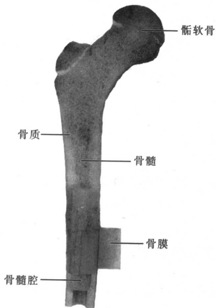
骨的构造
