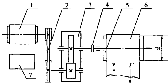
图 1.1 带式运输机
