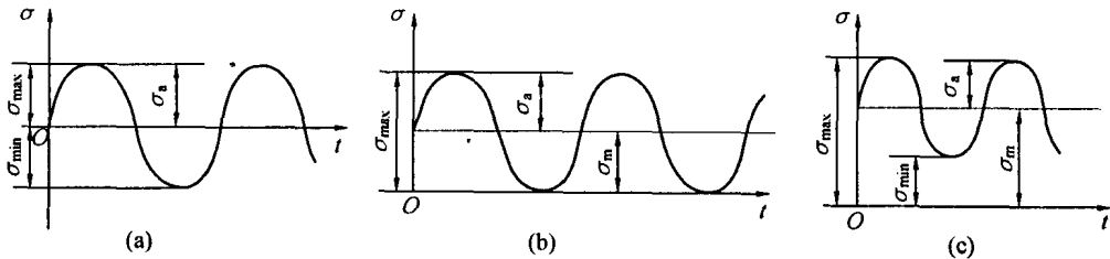
图 2.2 稳定循环变应力谱
