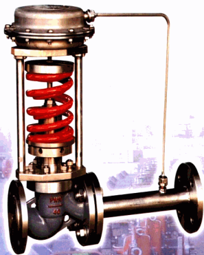
自力式压力调节阀
