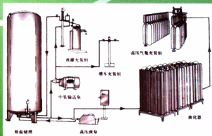
液态充装站
