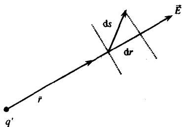
图 1.2 电场中移动电荷做的功
