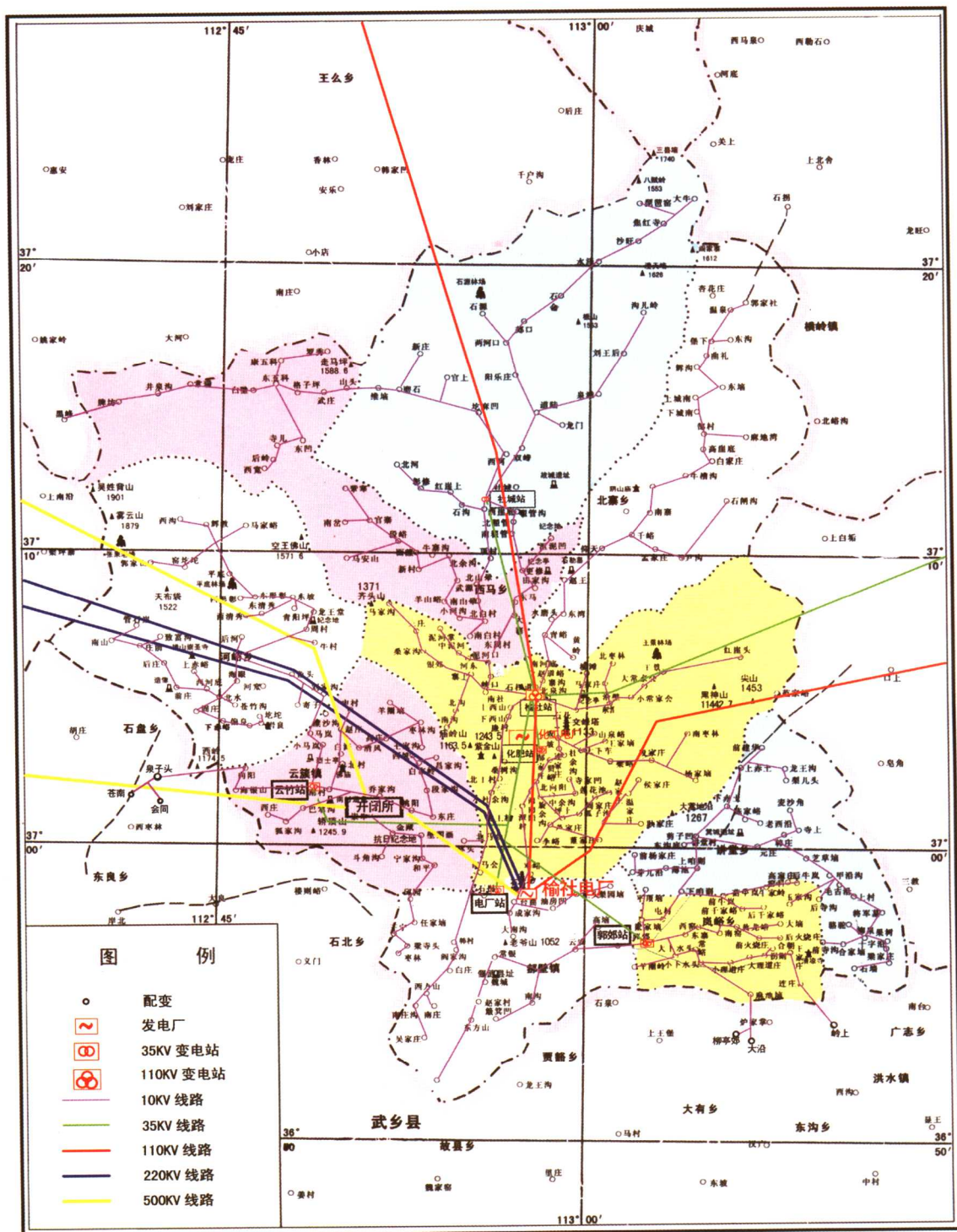
2004年榆社县输配电线路地理图
