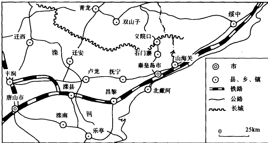
图 1-1 实习区交通位置图
