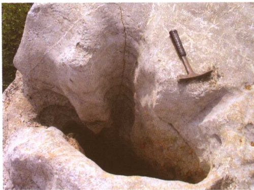
3. 沙锅店北东石灰岩中的落水洞
