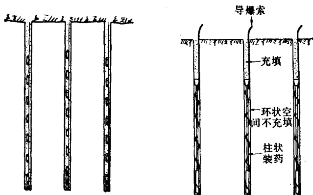
图 1-4 药卷交错排列均匀分布 图 1-5 炸药合理分布的柱状装药
