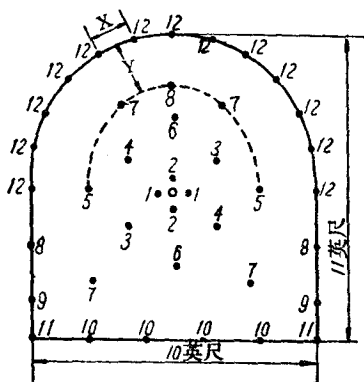
图 1-6 地下巷道典型段发顺序布置 (注: 图中Y比X大)
