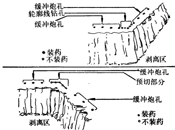
图 1-3 非线性工作面的缓冲爆破
