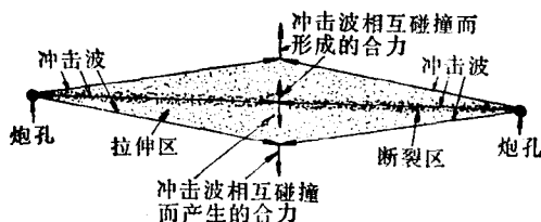
图 1-7 预裂爆破法的原理
