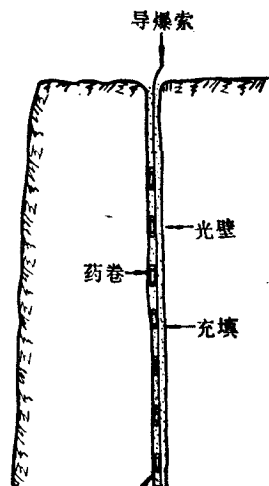
图 1-2 缓冲爆破法的炸药分布
