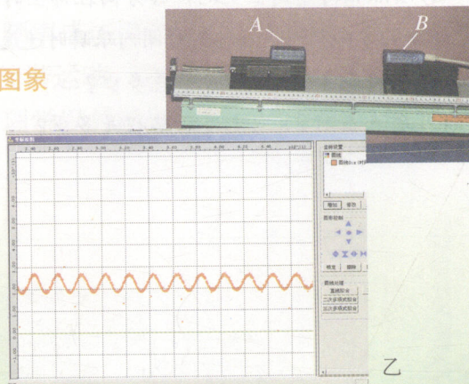
图 11.1-9 用传感器和计算机描绘简谐运动的图象
