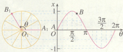
图 11.1-7 单位圆和正弦曲线
