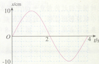
图 11.1-11 某质点的振动图象
