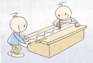
图 11.1-10 两人合作绘制振动图象
