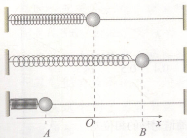
图11.3-2 弹簧振子的运动和它的能量
