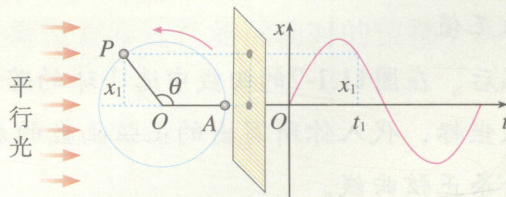
图 11.1-8 做匀速圆周运动的质点的投影的运动规律与简谐运动相同
