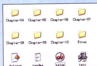
图 2 找到 TSCC
