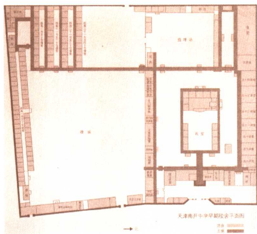
天津南开中学早期校舍平面图
