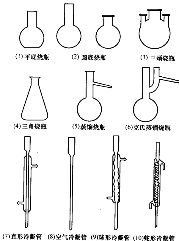
图 1-1 普通玻璃仪器（一）
