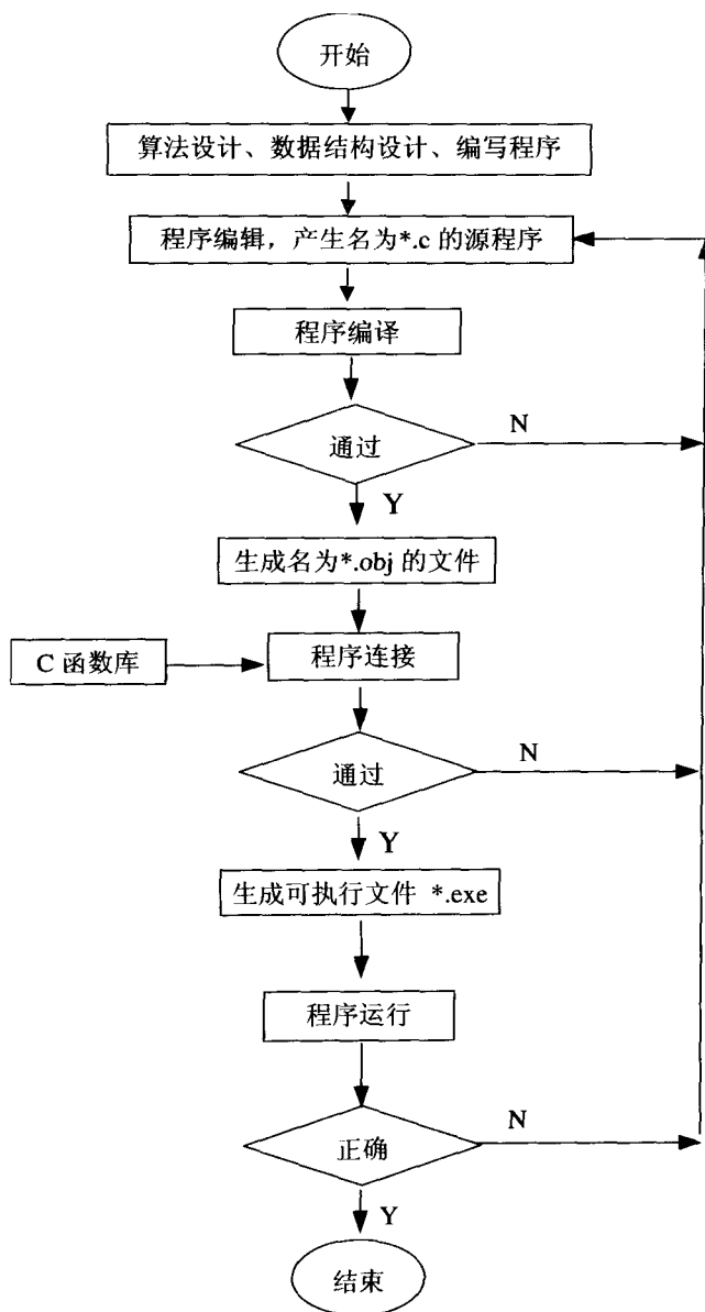
图 1.1 C 语言程序的开发过程
