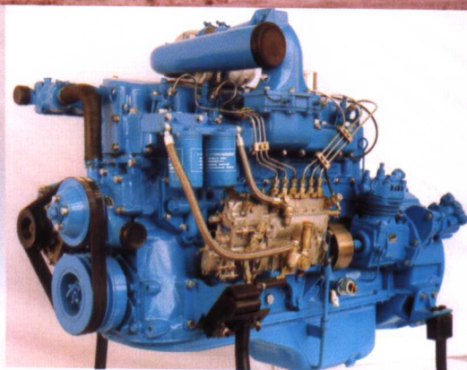
CA6110/125Z1A2 增压发动机
