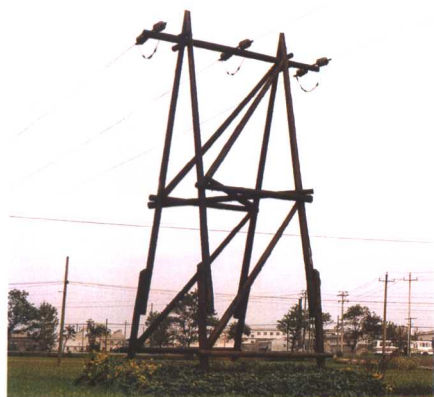
全省第一条35千伏输电线路(杭海线)
