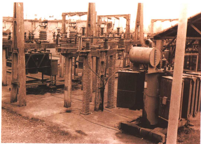
建于1957年的余杭首座35千伏临平变电所
