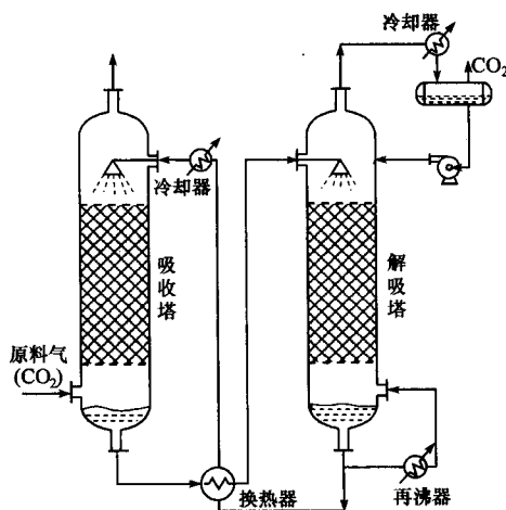
图 9.3 乙醇胺水溶液吸收 \text{CO}_2 流程
