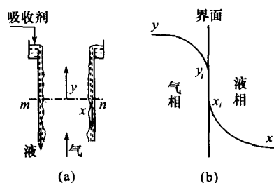
图 9.1 m-n 截面上溶质的浓度分布
