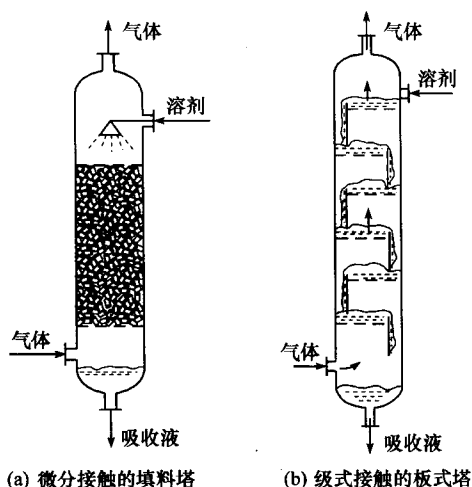
图 9.2 填料塔和板式塔
