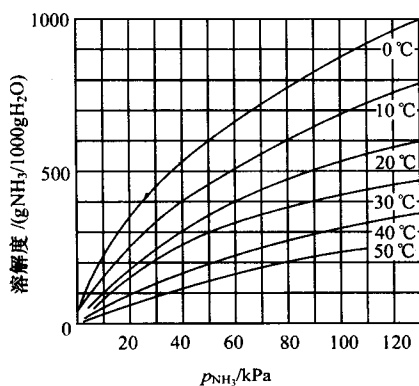
图 9.4 氨在水中的溶解度
