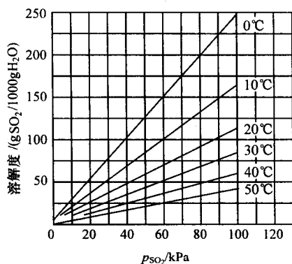
图 9.5 二氧化硫在水中的溶解度
