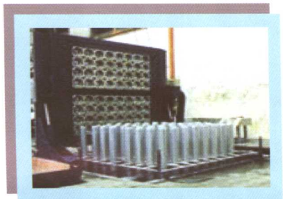
● 等水平热顶铸造机组
