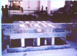
方锭铸造—同水平热顶铸造系统
