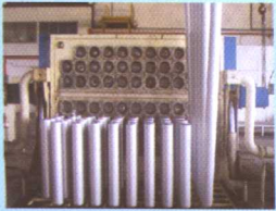
圆锭铸造—同水平热顶铸造系统
