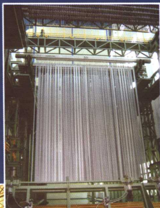
● 座地立式电泳炉
