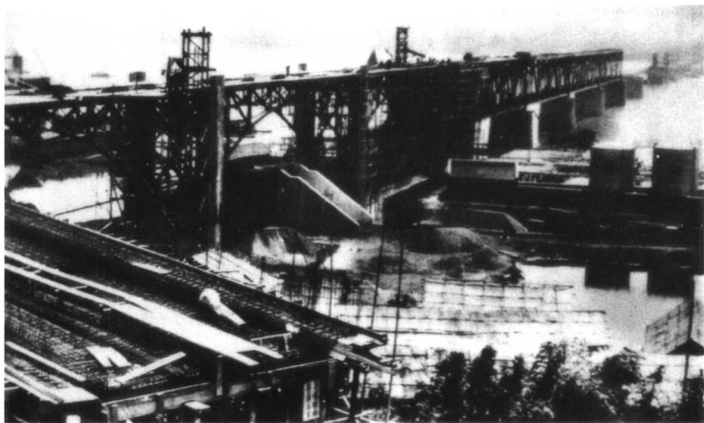
兴建中的钱塘江大桥。该桥 1935 年开工,1937 年建成。
