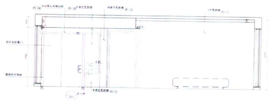
客厅立面图 1
