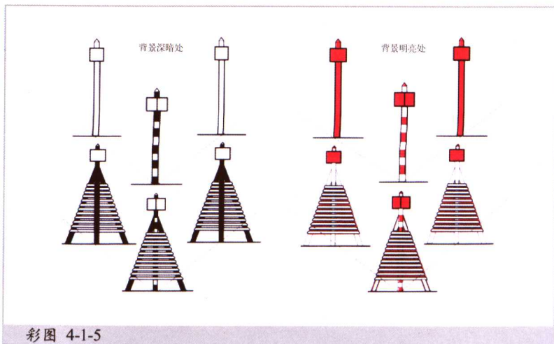
首尾导标
