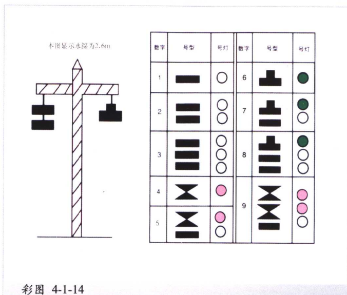
水深信号标
